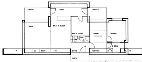
PLAN REZ DE CHAUSSEE
